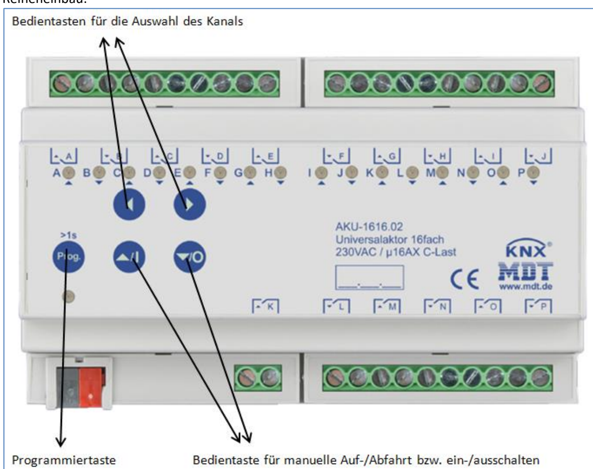
Abbildung 4: Übersicht Hardwaremodul
