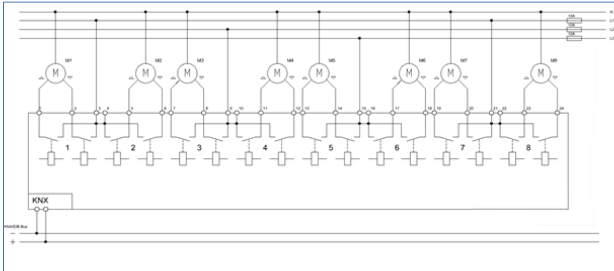
Abbildung 1: Anschlussbeispiel Jalousieaktor
